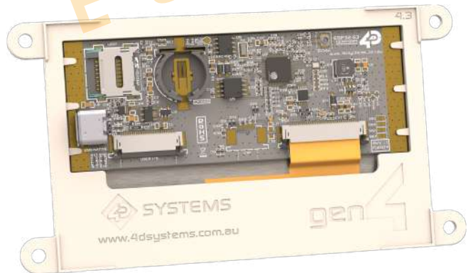
gen4-ESP32Q-43T Rear
