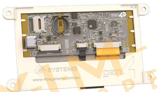
gen4-ESP32Q-43CT Rear
