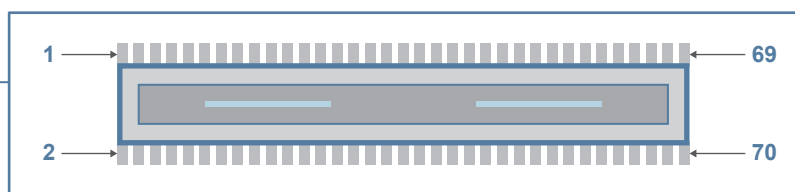
DF40C-70DP-0.4V(51)
