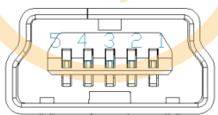
Figure 11: Mini USB Connector
