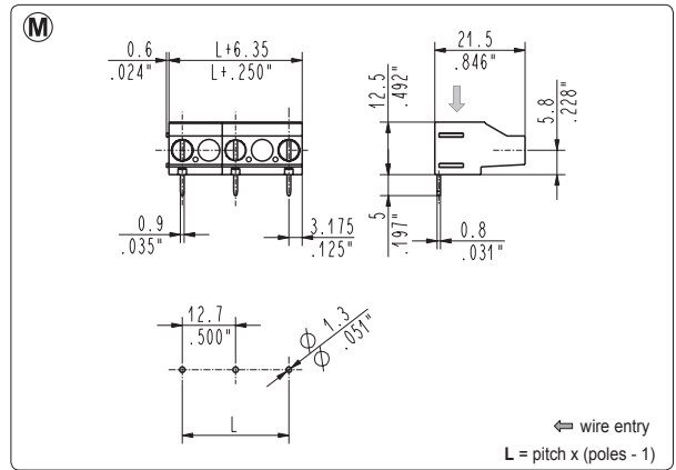
MSP_09U 90°, modular
