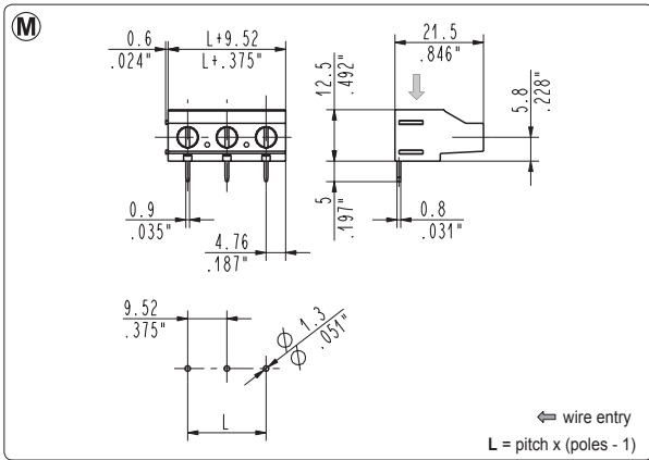
MSP_09N 90°, modular
