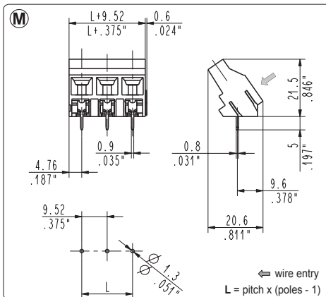
MSP_04N 35°, modular
