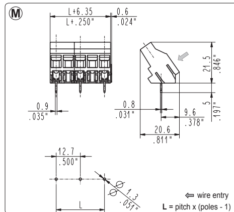
MSP_04U 35°, modular
